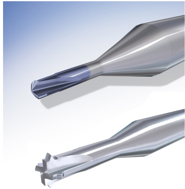
Extrem präzise Mikrowerkzeuge von Zecha: Oben: Ein kurzer, gerade verzahnter Einschneider, Torx-Fräser, Serie 471 oder der Gewindewirbler, Serie 462.
